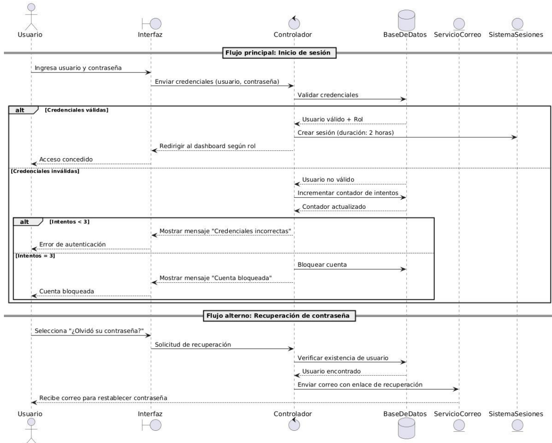
Diagrama de Secuencia – Historia de usuario 00: Inicio
