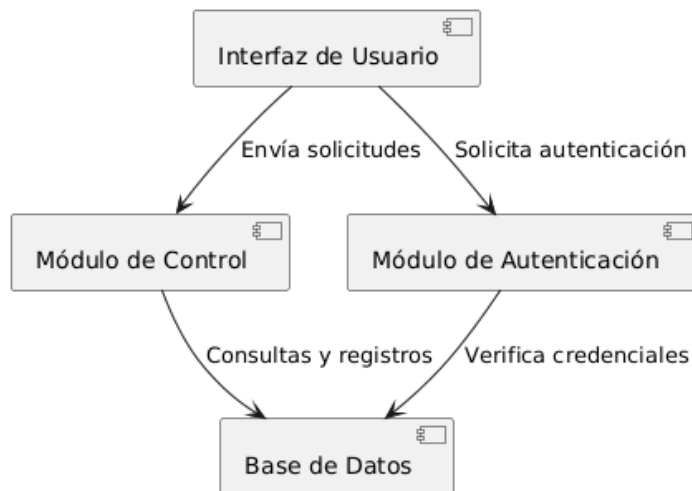
Diagrama de Componentes– Historia de usuario 02: Registro
