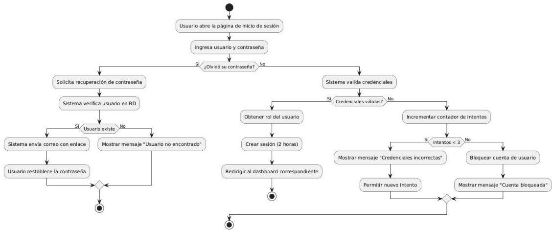
Diagrama de actividad – Historia de usuario 00: Inicio Sesión
