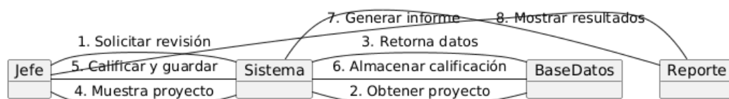
Diagrama de Comunicación: Calificación de Proyecto
