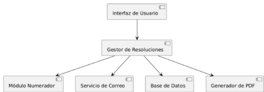
Diagrama de Componentes: Gestión de Resoluciones Directorales
