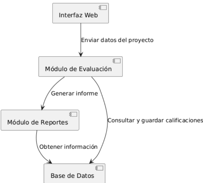
Diagrama de Componentes: Sistema de Evaluación
