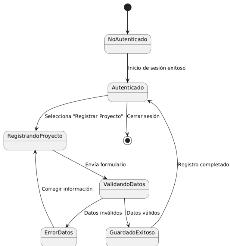
Diagrama de Estado – Historia de usuario 02: Registro
