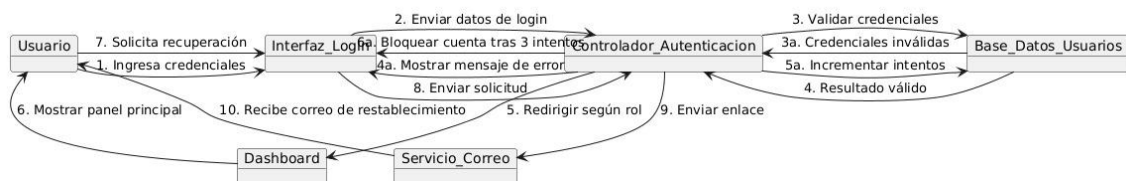
Diagrama de Comunicación - Inicio de Sesión
